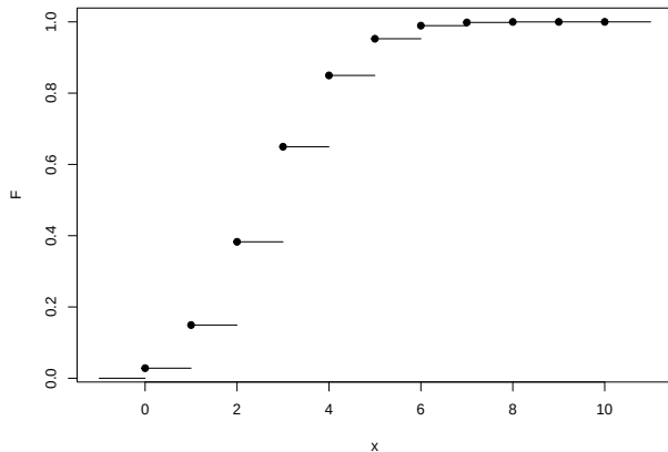
Abbildung 2: Verteilungsfunktion B(10, 0.3)
